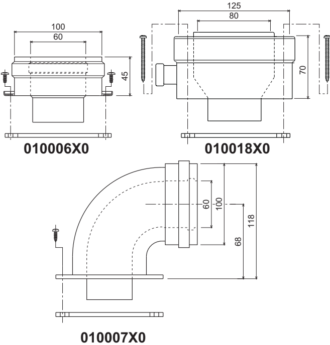
fig. 11 - Accesorios iniciales para conductos coaxiales
