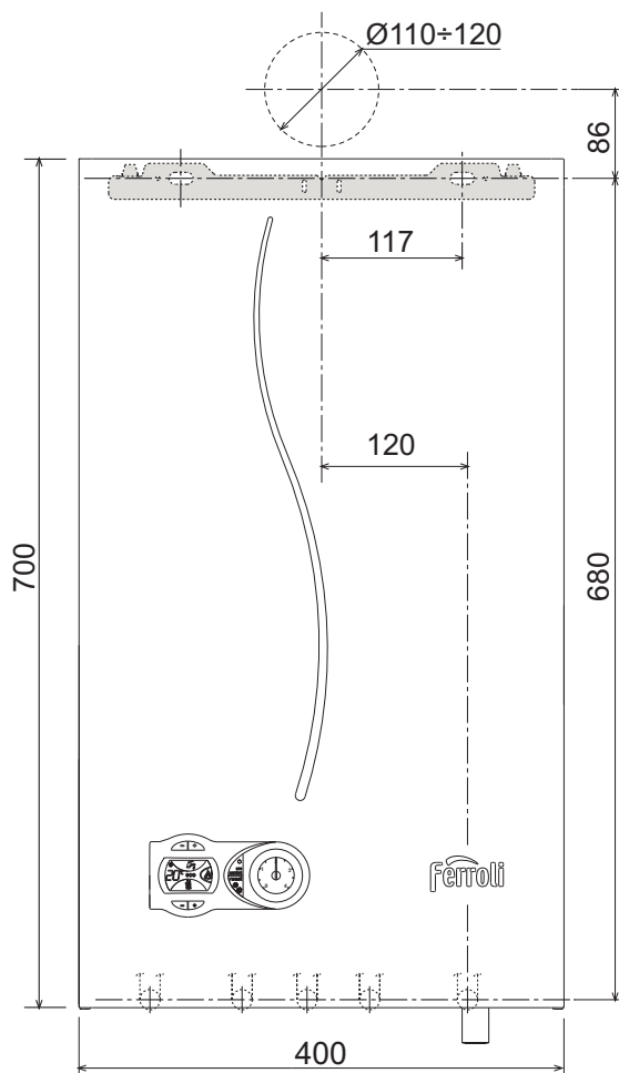
fig. 18 - Vista frontal
