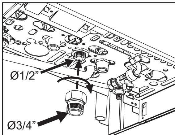
fig. 8 - Reducción de 1/2" a 3/4"
