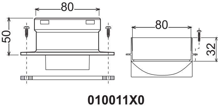
fig. 13 - Accesorio inicial para conductos separados
