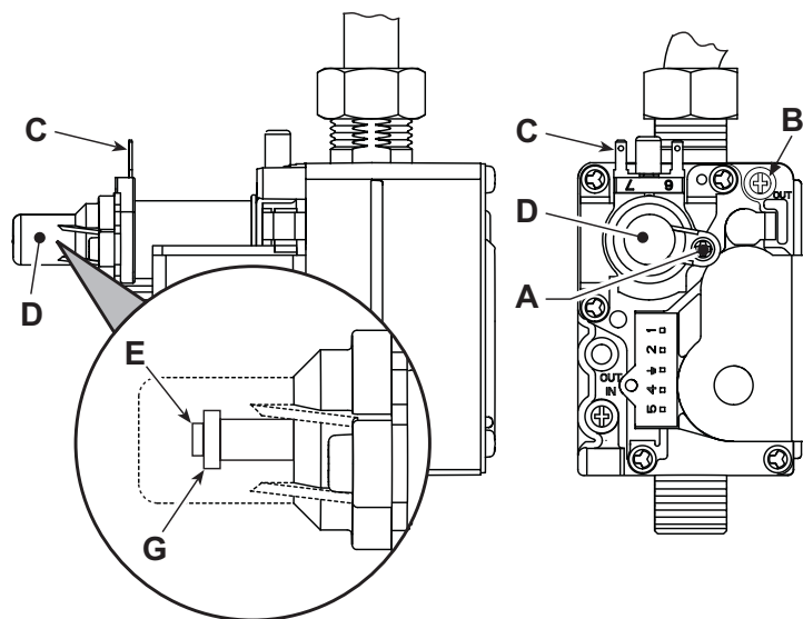
fig. 16 – Válvula de gás
