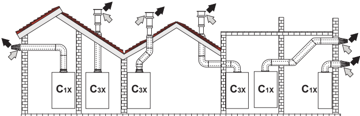
fig. 10 - Ejemplos de conexión con tubos coaxiales ( ➡ = aire / ➡ = humos )
