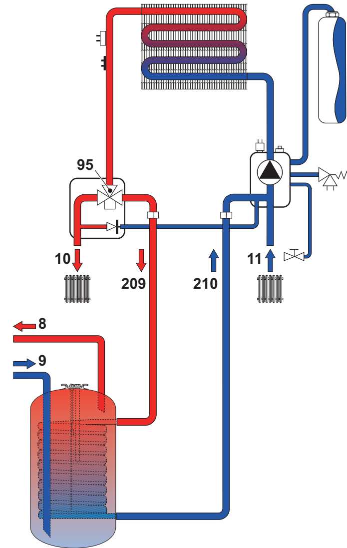
fig. 7 - Esquema de conexión a un termostanque externo
