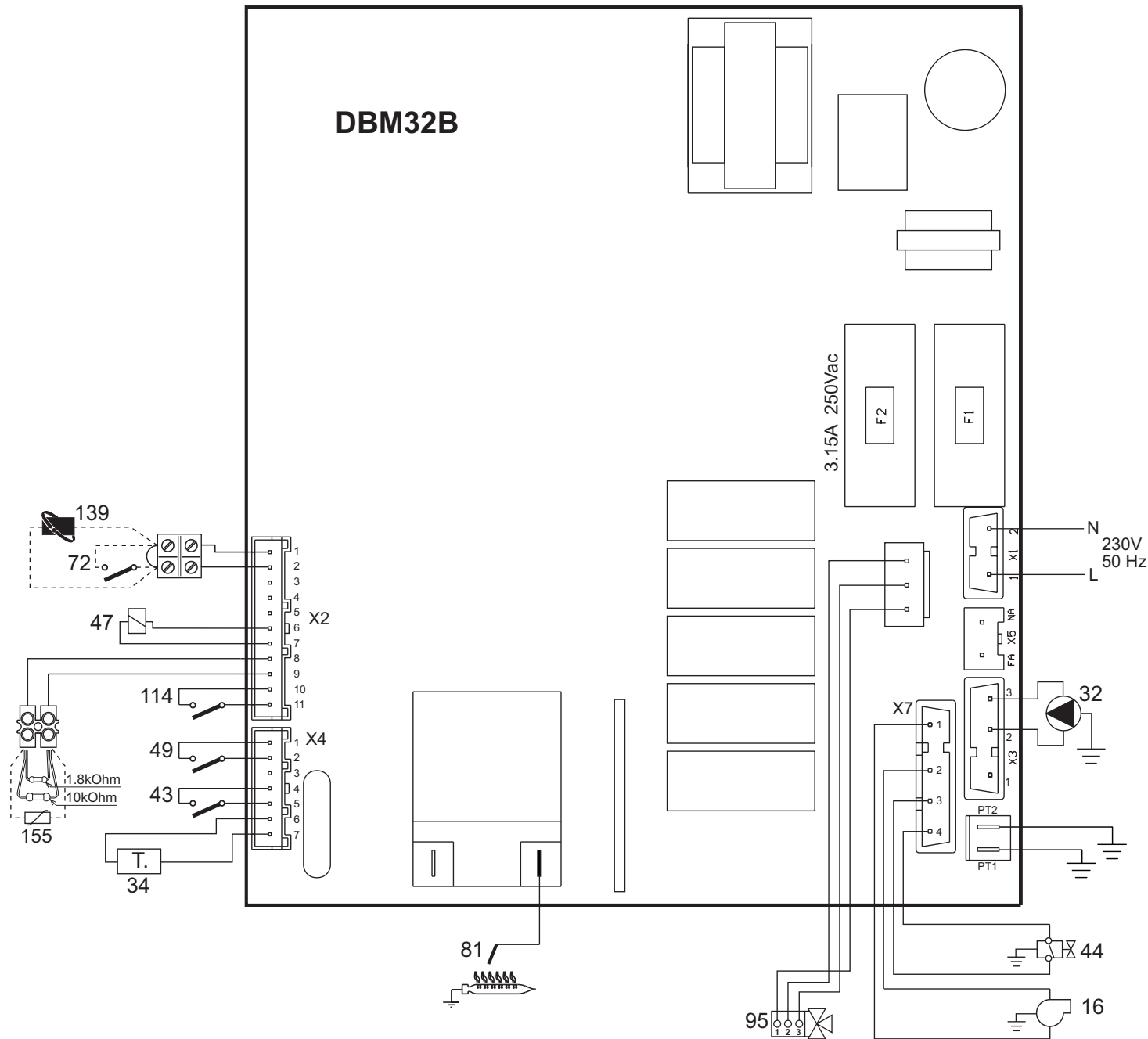
fig. 24 – Esquema eléctrico
