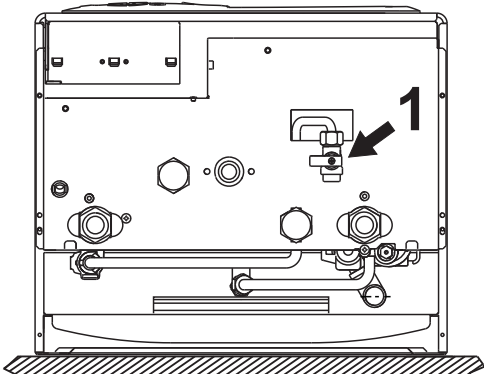
fig. 6 – Torneira de enchimento
