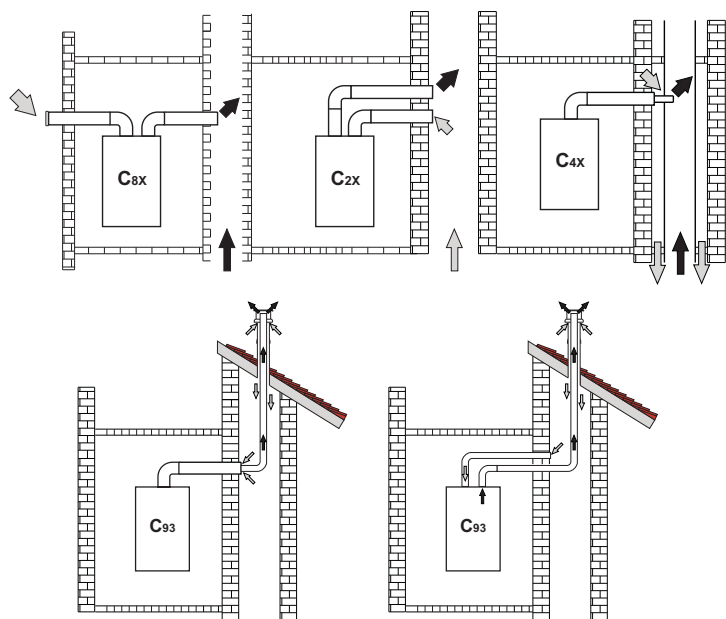
fig. 14 – Exemplos de ligação a tubos de evacuação de fumos (Ar/ = Fumos)
